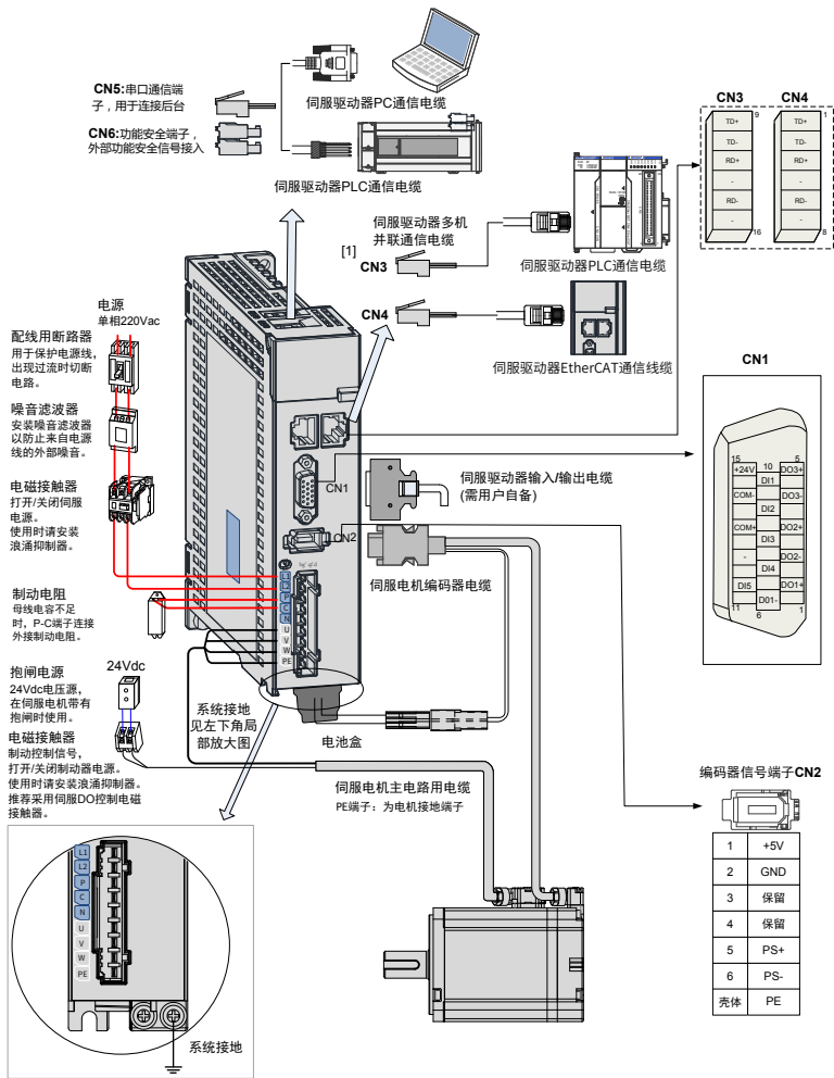
图 1-5 单相 220V 系统配线图示例
