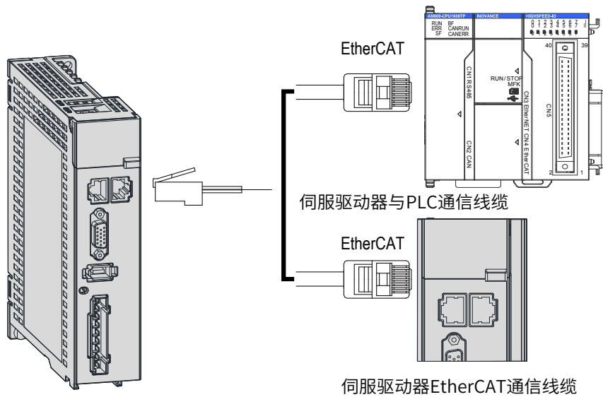
图 3-24 通信配线示意图
