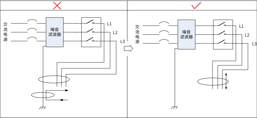
图 3-29 噪声滤波器地线与输出配线分离走线示意图
