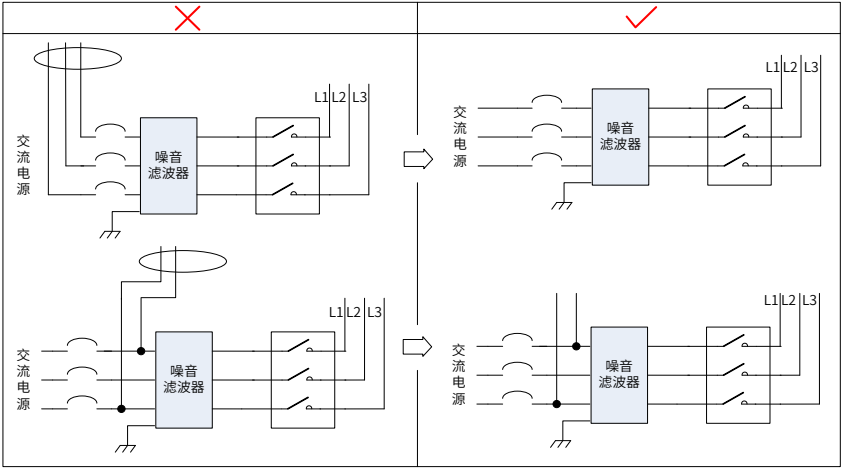
图 3-28 噪声滤波器输入与输出配线分离走线示意图
