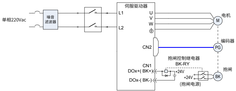
图 4-3 抱闸配线图
