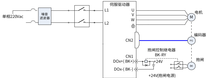
图 3-22 抱闸配线图
