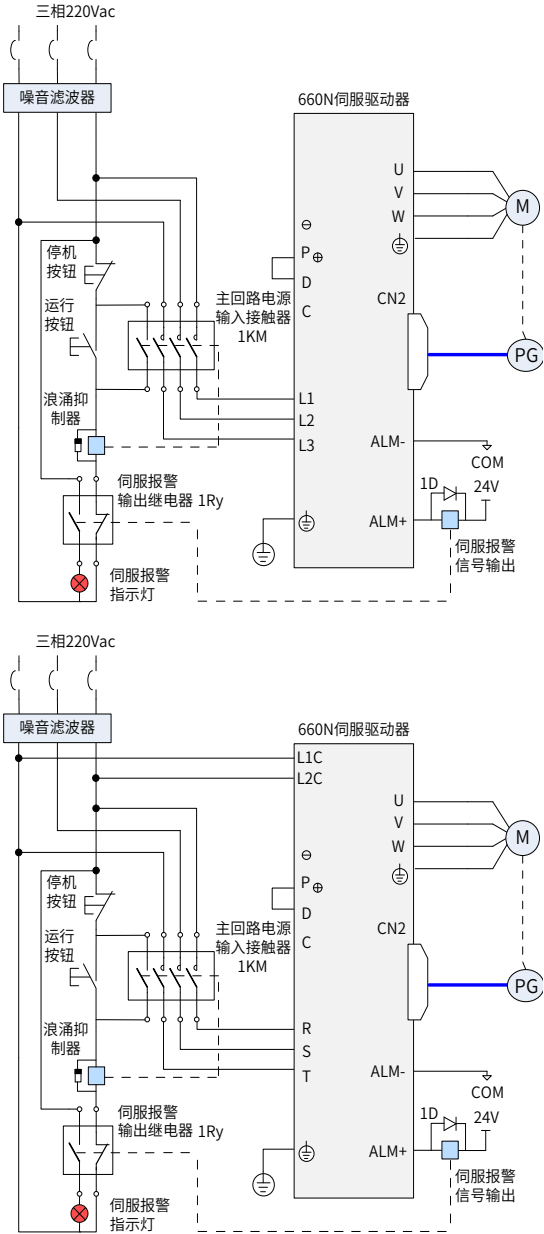
图 3-12 三相 220V 主电路配线
