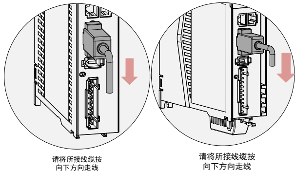
图 2-5 伺服驱动器线缆走线要求示意图
