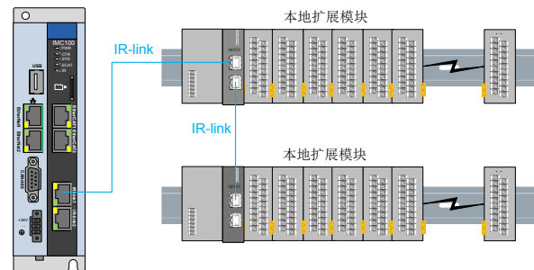
图 2-4 IRlink 通讯模块的组网示意图
