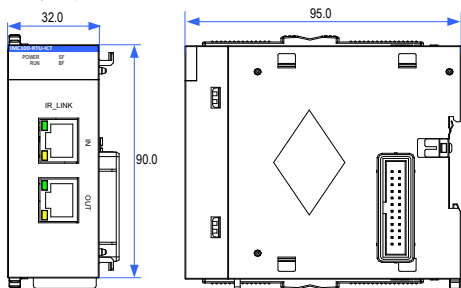
图 2-2 IRlink 通讯模块尺寸图 (单位: mm)
