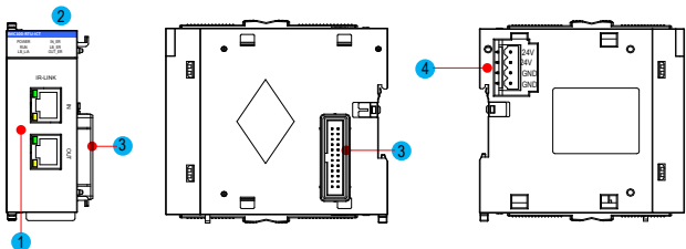
图 2-3 IRlink 通讯模块端口示意图
