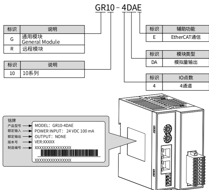
图1 型号与铭牌说明
