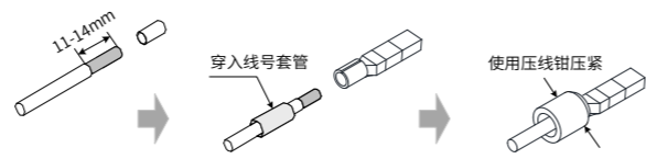
图3 线缆制作示意
