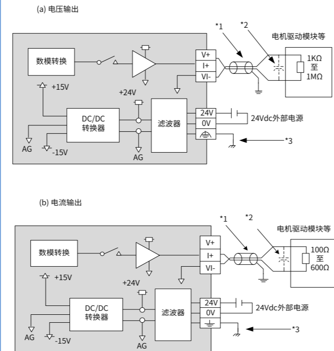
图4 模块接线图
