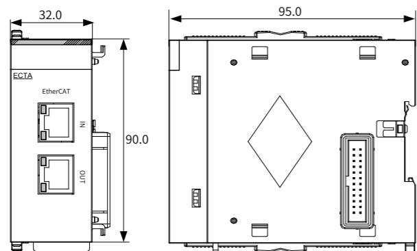
图3 安装尺寸 (单位: mm)
