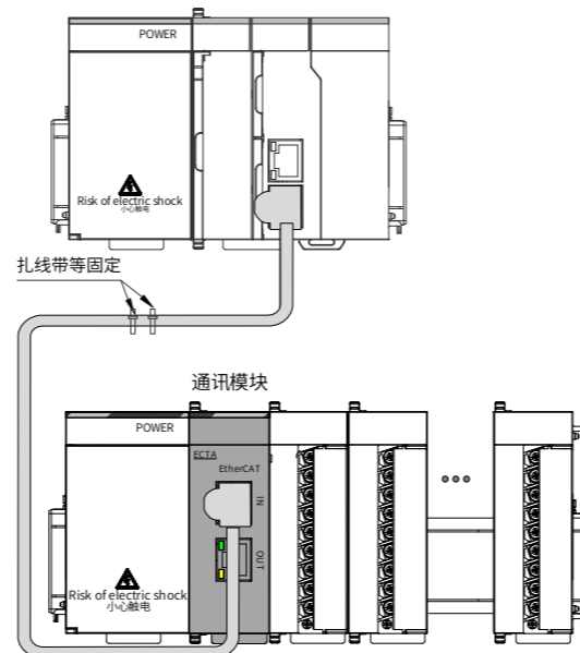
图8 通讯线缆在靠近设备侧需做必要固定
