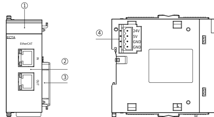
图2 模块接口示意
