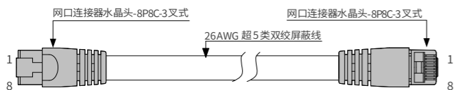
图5 EtherCAT 网线制作要求
