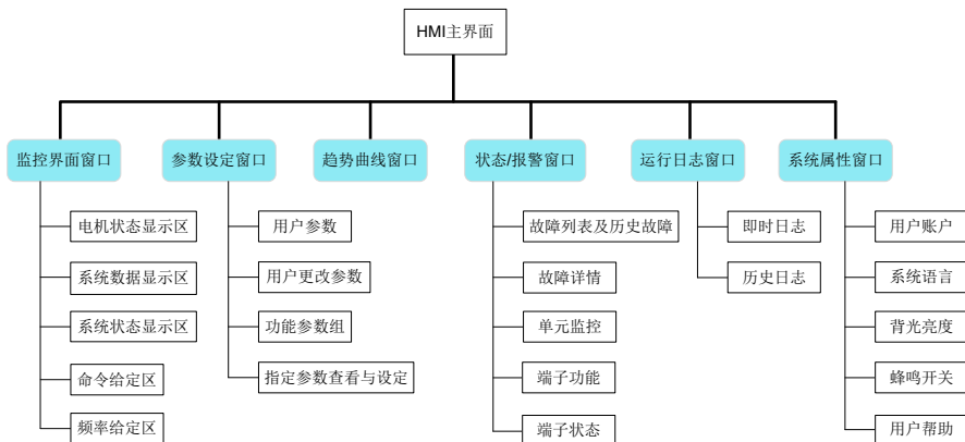
图 6-1 HMI 功能示意框图
