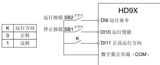
图 8-5 三线式控制模式 2
