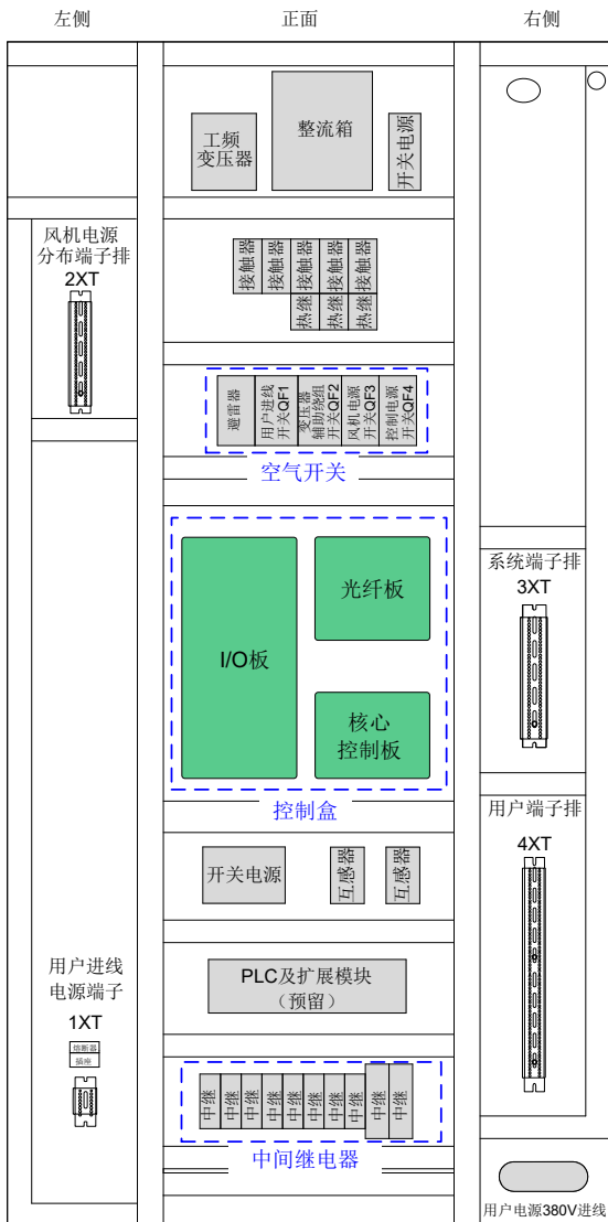
图 3-25 控制盘器件布局图
