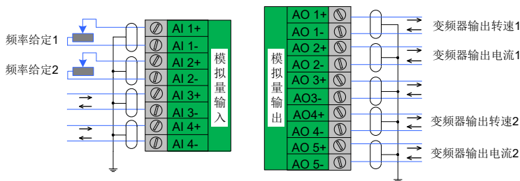
图 3-29 模拟量输入输出端子接线
