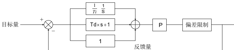
图 8-7 过程 PID 原理框图
