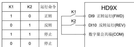
图 8-2 两线式模式 1
