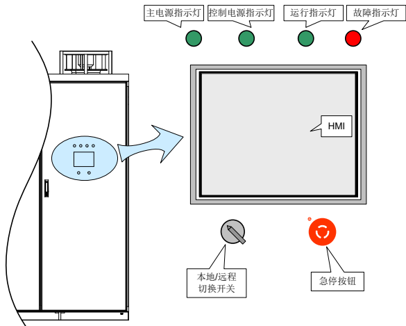
图 5-1 控制柜面板示意图
