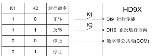
图 8-3 两线式模式 2
