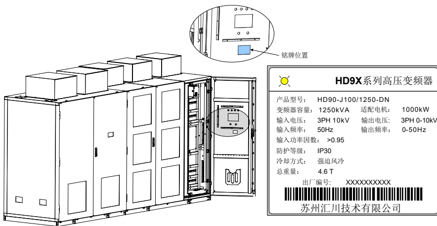
图 2-2 铭牌信息
