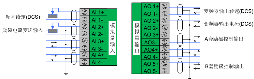
图 3-35 模拟量输入输出端子接线
